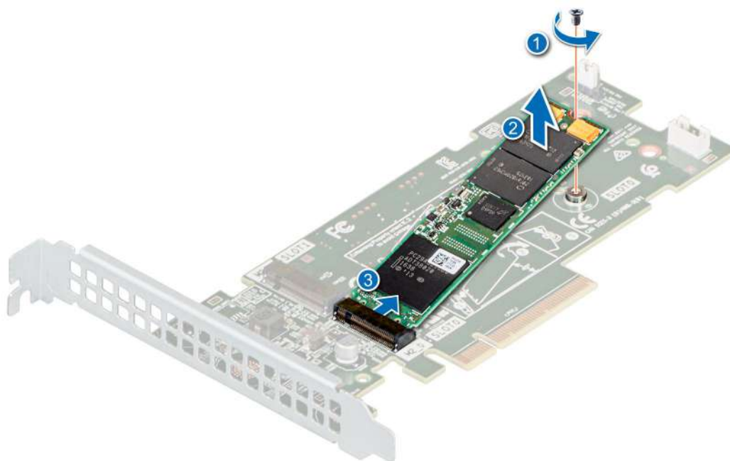
Ilustración 59. Extracción del módulo M.2 SSD
