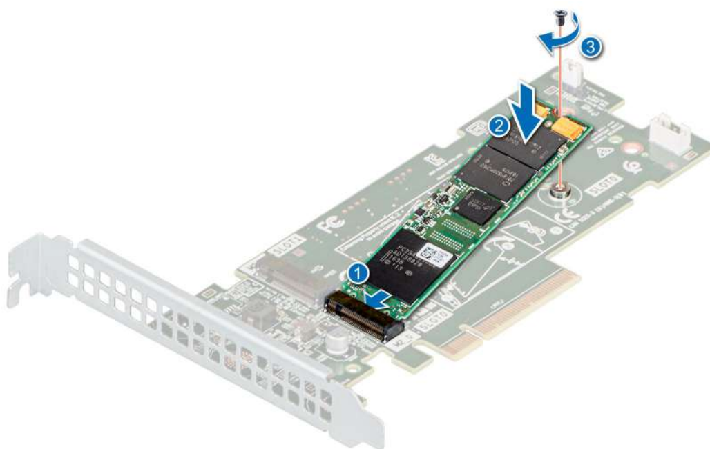
Ilustración 60. Instalación del módulo M.2 SSD
