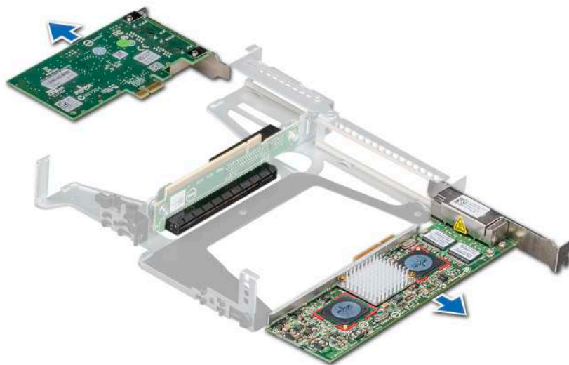
Ilustración 41. Extracción de la tarjeta de expansión del soporte vertical para tarjetas de expansión
