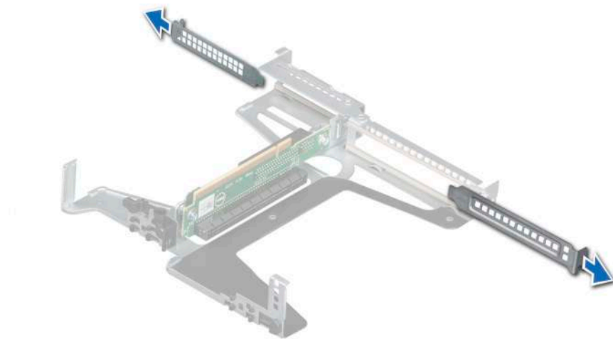
Ilustración 43. Extracción de la tarjeta de expansión de relleno
