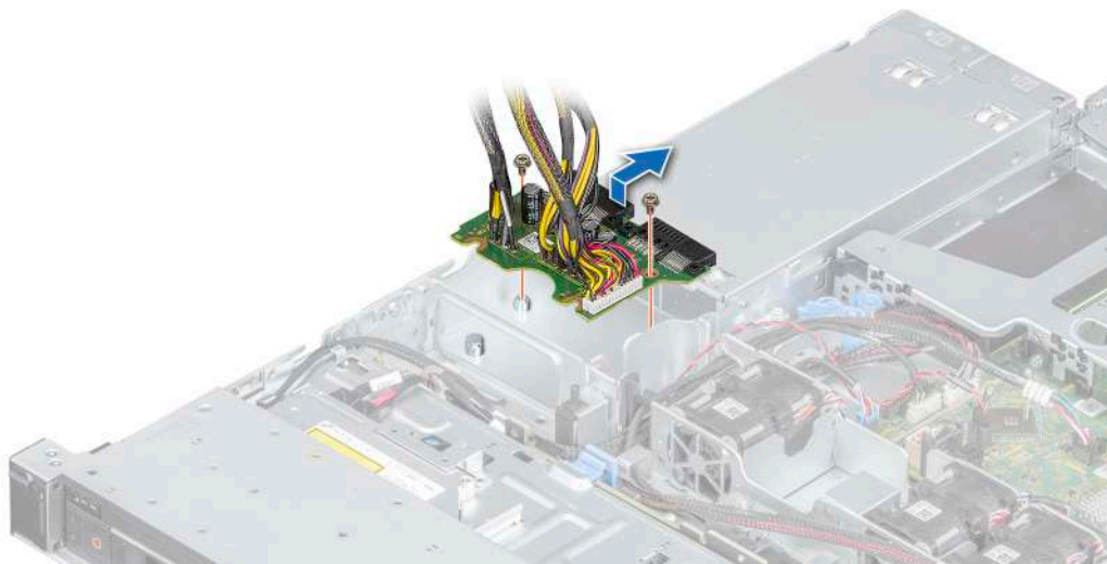
Ilustración 72. Extracción de la placa de distribución de alimentación
