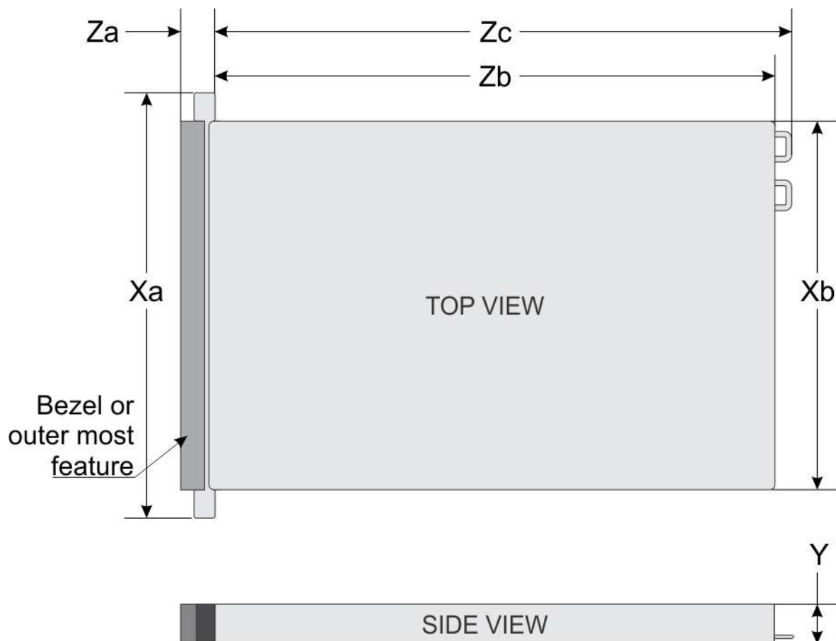
Ilustración 83. Dimensiones del chasis
