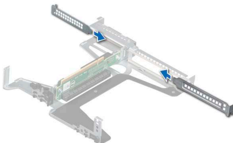
Ilustración 42. Instalación de la tarjeta de expansión de relleno
