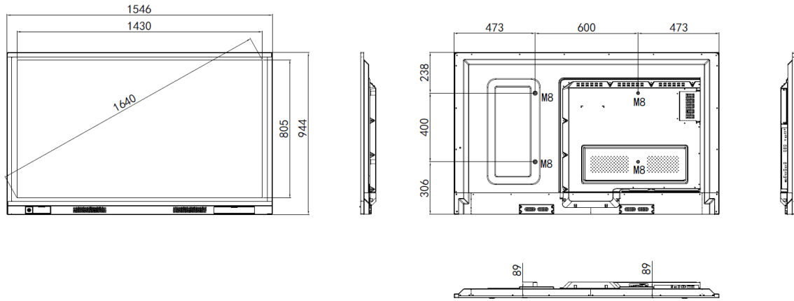
65" Dimensions
