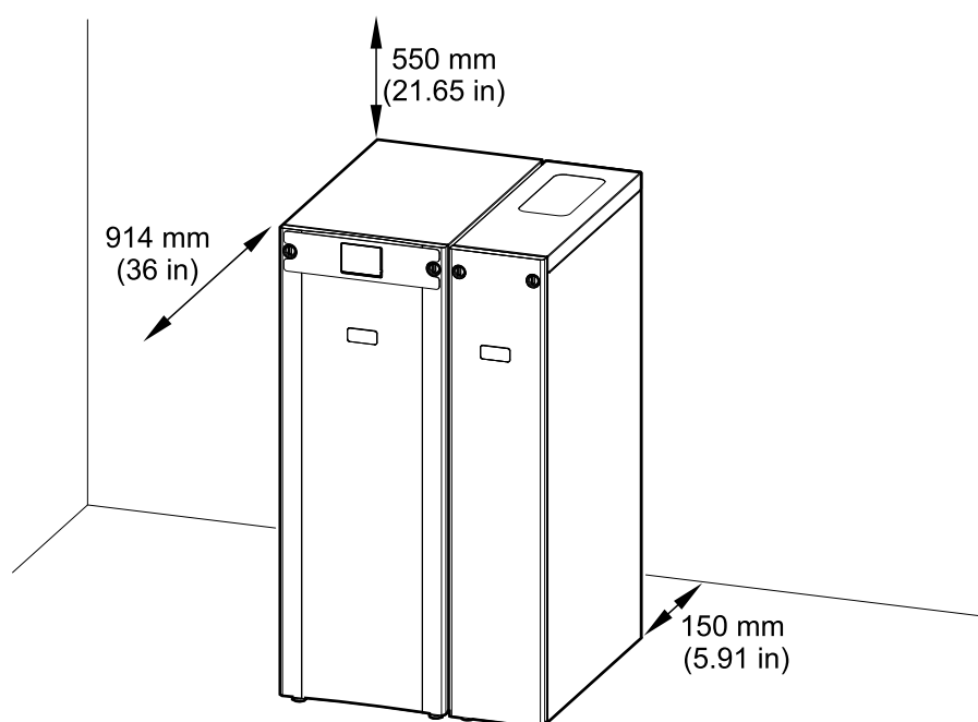
Vue avant de l'ASI et de l'armoire de bypass de maintenance
