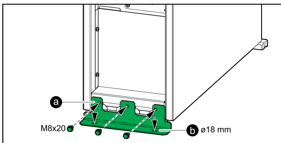
Vue avant de l'armoire de bypass de maintenance
