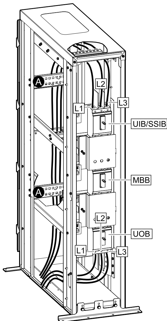
Armoire de bypass de maintenance sans boîtier de câblage
