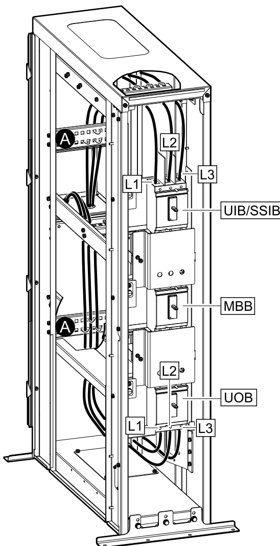
Armoire de bypass de maintenance avec boîtier de câblage
