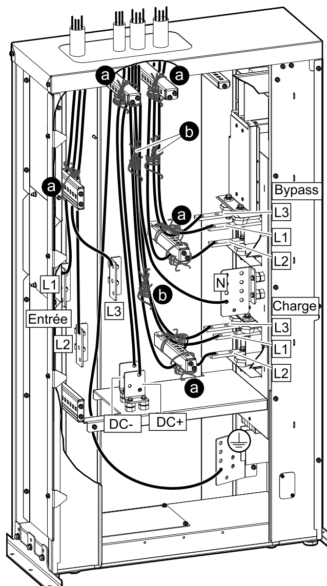
Vue du côté gauche de l'armoire de bypass de maintenance - Alimentation secteur double
