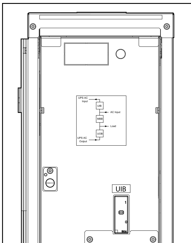
Vue avant de l'armoire de bypass de maintenance, alimentation secteur simple
