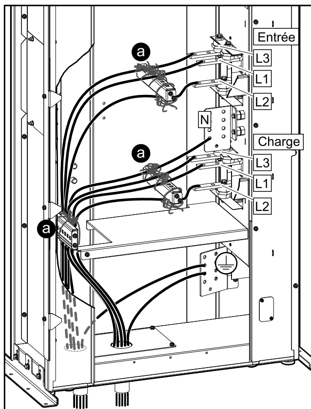
Vue du côté gauche de l'armoire de bypass de maintenance - Alimentation secteur simple
