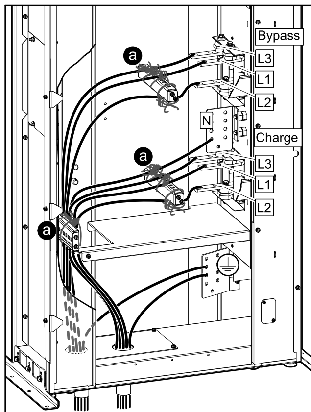
Vue du côté gauche de l'armoire de bypass de maintenance - Alimentation secteur double
