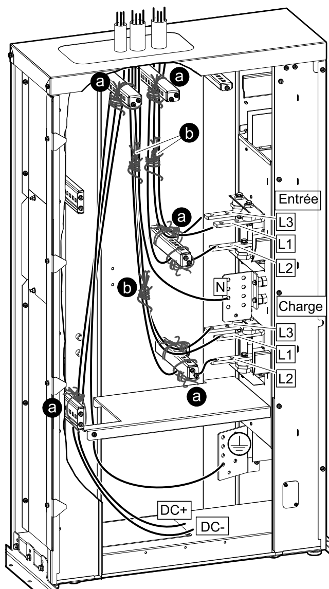
Vue du côté gauche de l'armoire de bypass de maintenance - Alimentation secteur simple
