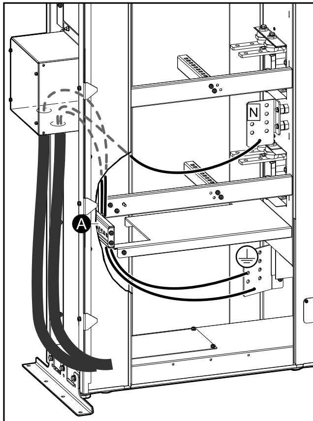
Vue du côté gauche de l'armoire de bypass de maintenance avec boîtier de câblage
