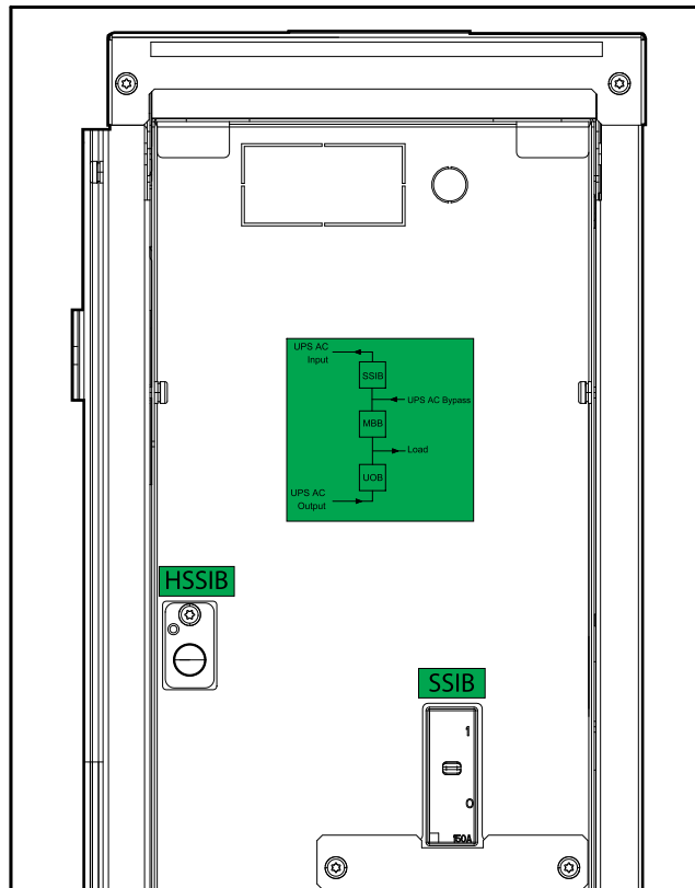
Vue avant de l'armoire de bypass de maintenance, alimentation secteur double
