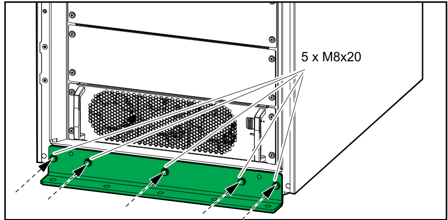
Vue avant (avec feuille de calage)
