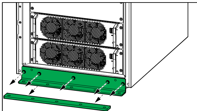
Vue avant de l'ASI (avec feuille de calage)
