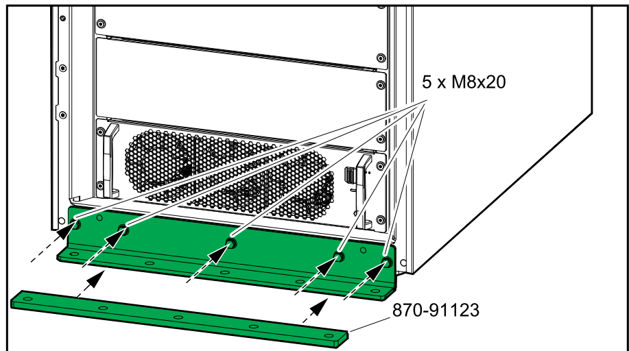
Vue avant (sans feuille de calage)
