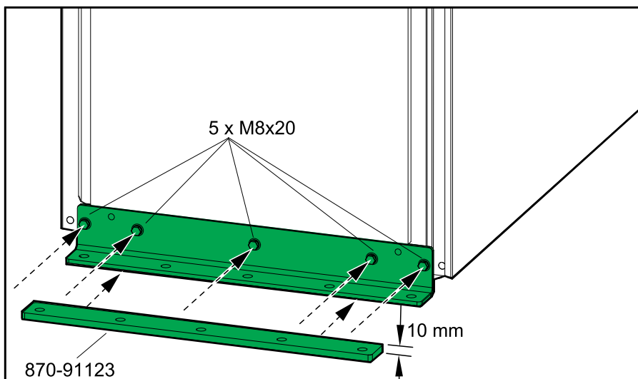
Vue arrière (avec feuille de calage)
