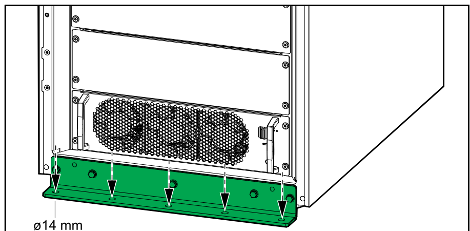
Vue avant (sans feuille de calage)
