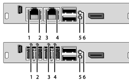
CON Module
