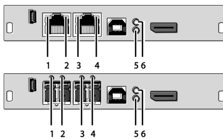
CPU Module
