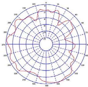
H-Plane (2400MHz)
