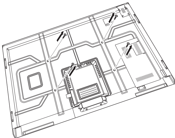
AP-WALLMNT-2
