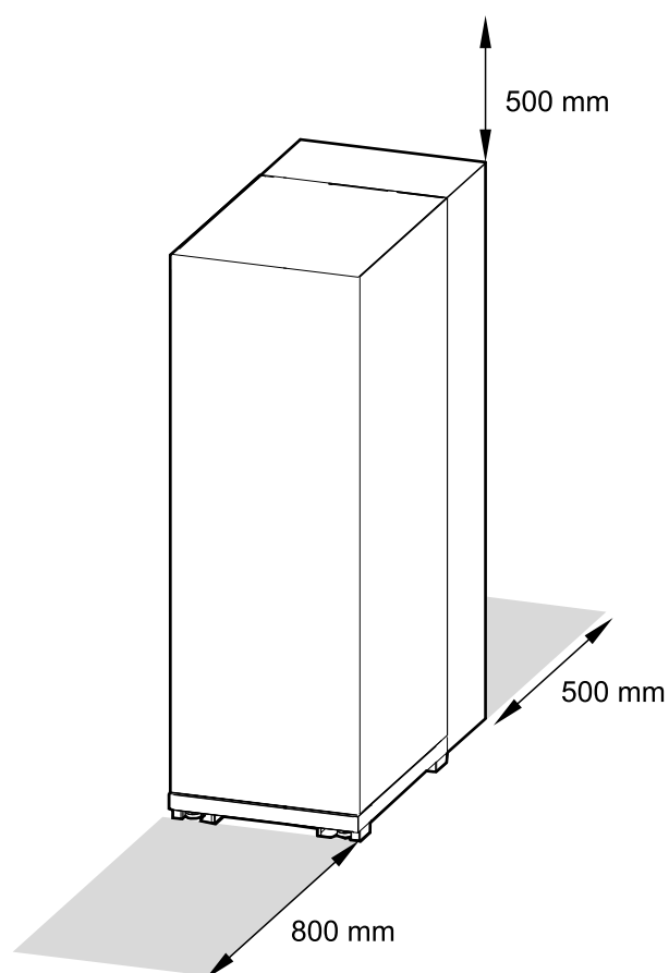
ASI avec adaptateur de profondeur
