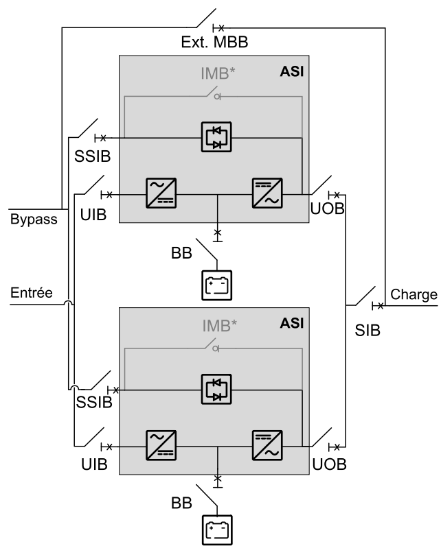
Système parallèle - Alimentation secteur double (un commutateur interne)
